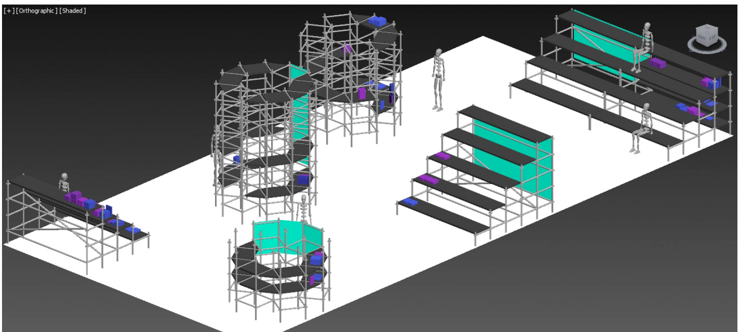
Τριδιάστατες ψηφιακές απεικονίσεις της προκαταρκτικής σχεδιαστικής πρότασης: τυπολογικές δομές τύπου αμφιθεάτρου και αντιπαραβάλλονται με την ανθρώπινη κλίμακα. Οι πράσινες επιφάνειες αντιπροσωπεύουν ενδεχόμενες επιφάνειες "τα μπλε και μοβ στοιχεία εκθεσιακά δείγματα."
