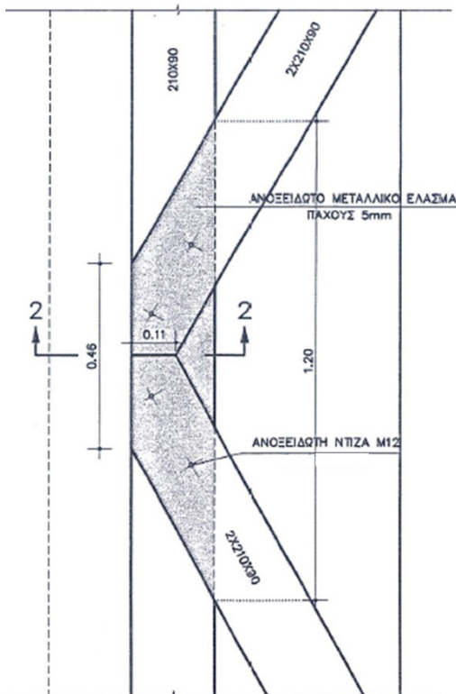
Σχήμα 3: Λεπτομέρεια μεταλλικών στοιχείων συνδέσεων - «Τύπος Λ9»
