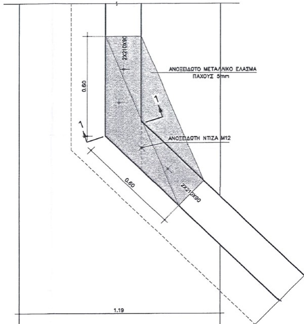
Σχήμα 3: Λεπτομέρεια μεταλλικών στοιχείων συνδέσεων - «Τύπος Λ9»
