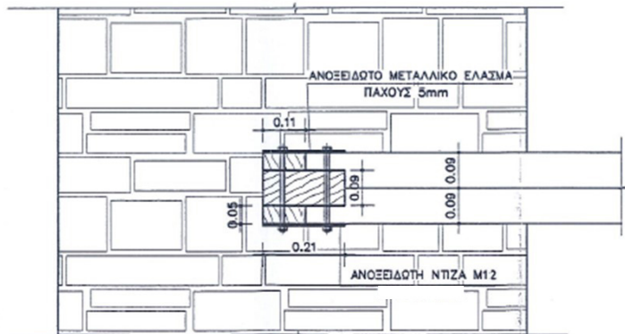
ΤΟΜΗ 2-2
