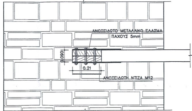
ΤΟΜΗ 1-1
