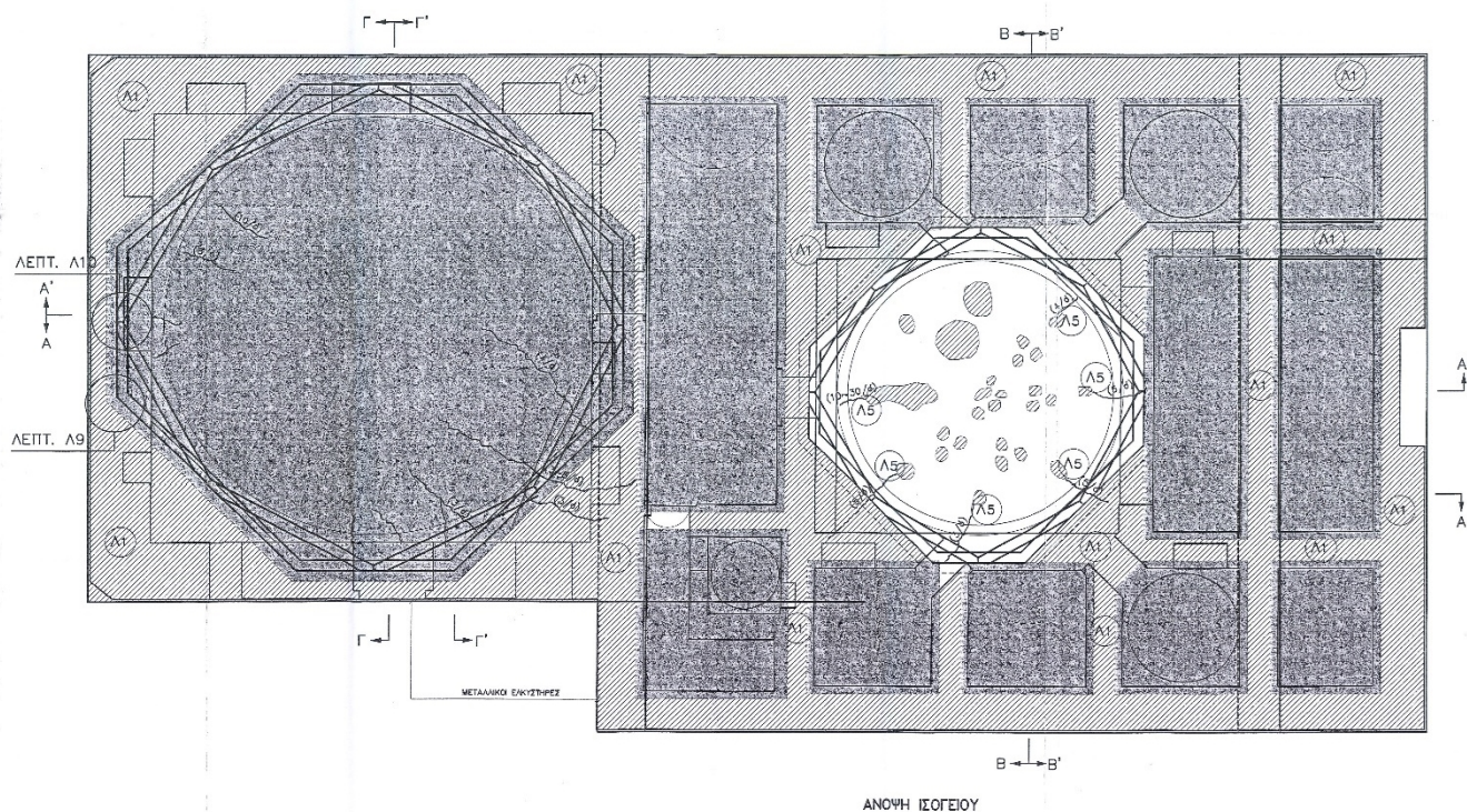
Σχήμα2: Κάτοψη - Ξύλινοι ελκυστήρες στα τύμπανα των τρούλων.
