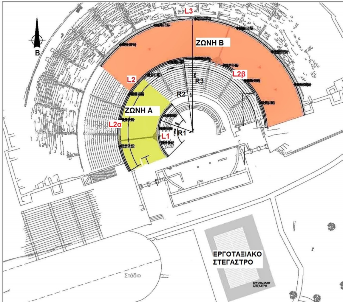
Τοποθέτηση γερανοτροχιάς στις δύο θέσεις εργασίας
