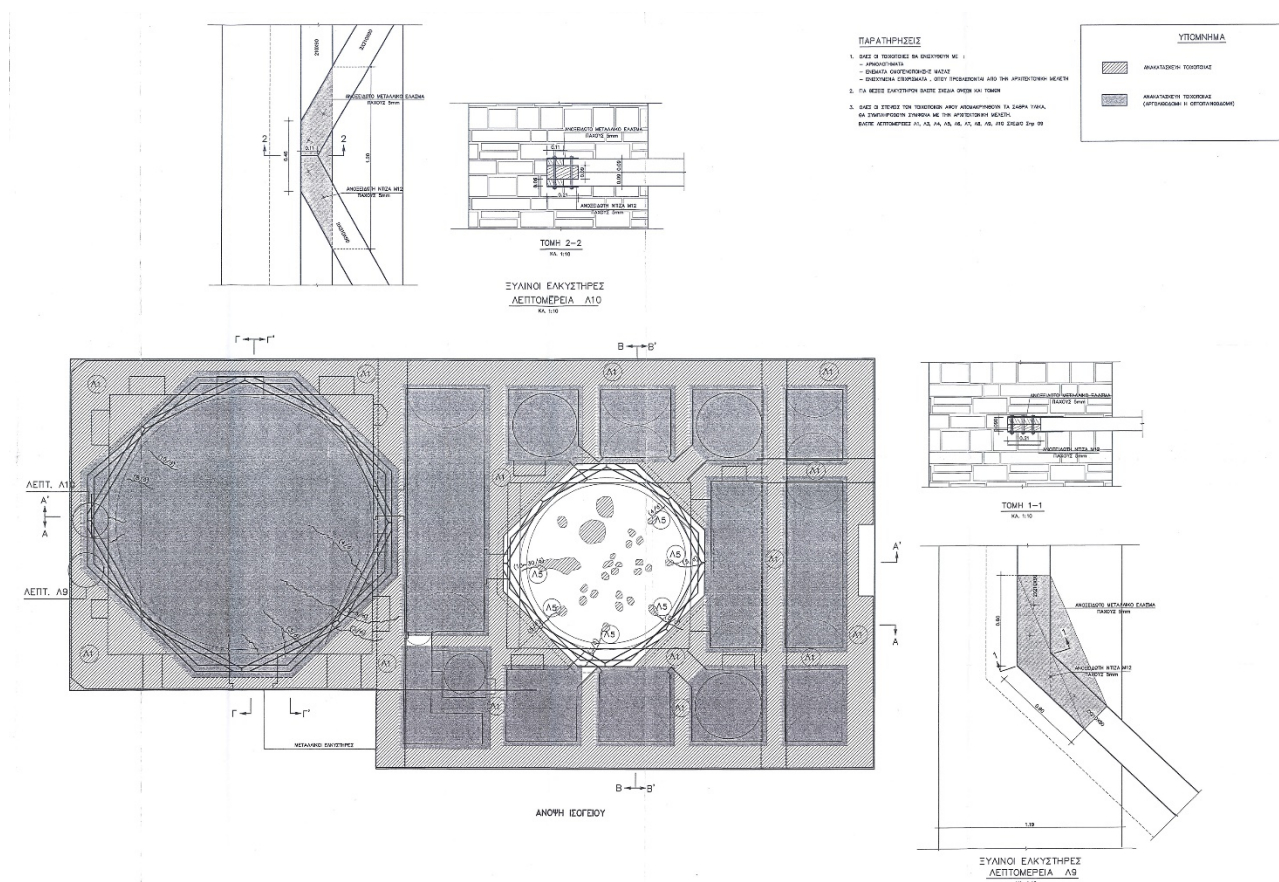
Σχήμα1: Κάτοψη – Ξύλινοι ελκυστήρες στα τύμπανα των τρούλων
