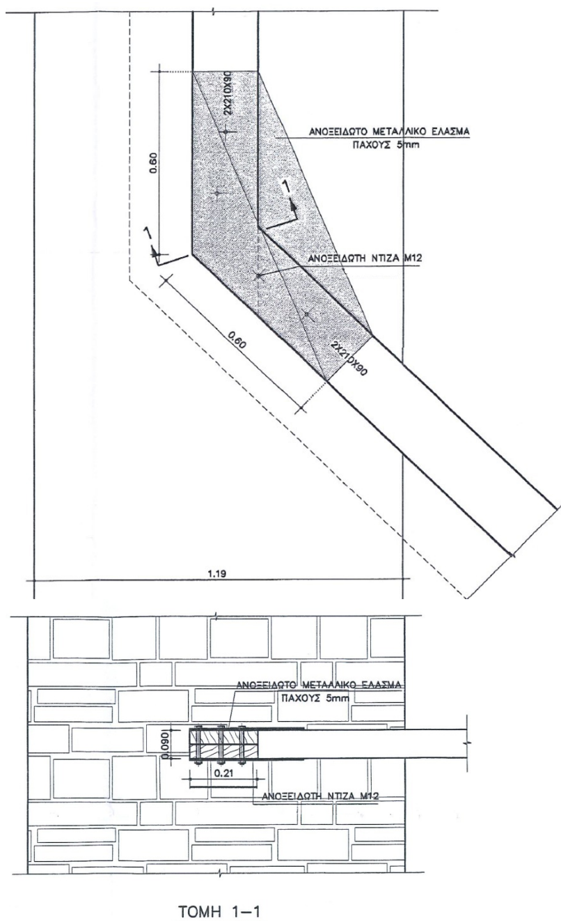
Σχήμα3: Λεπτομέρεια μεταλλικών στοιχείων συνδέσεων - τύπος Λ9
