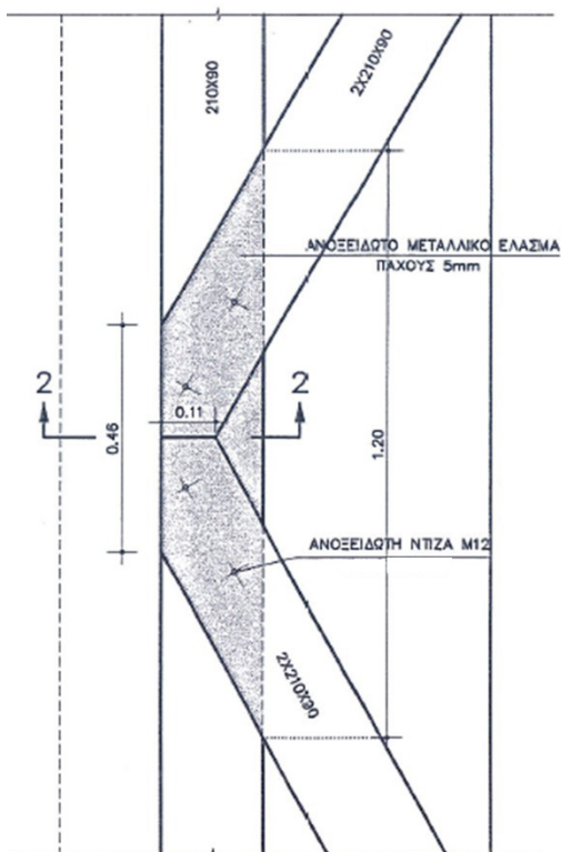
Σχήμα2: Λεπτομέρεια μεταλλικών στοιχείων συνδέσεων - τύπος Λ10
