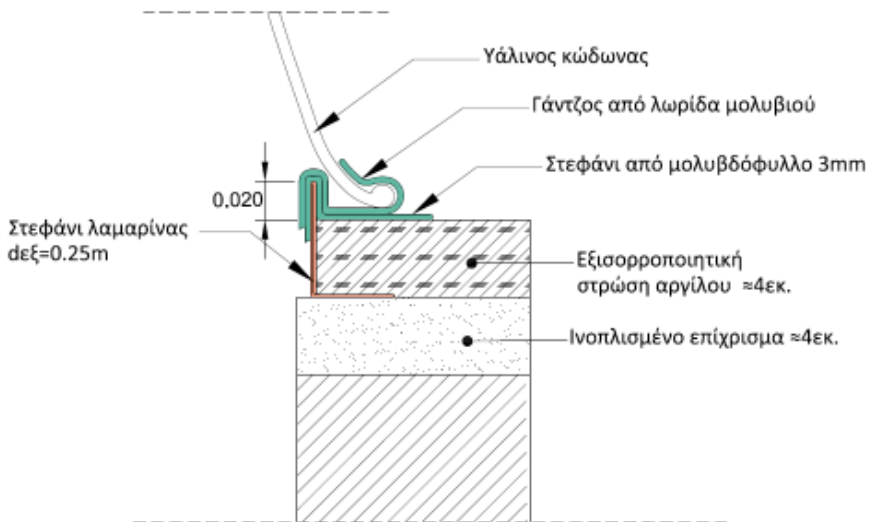
Εικόνα 6: Λεπτομέρεια στερέωσης υάλινου κώδωνα (τύπος Α)
