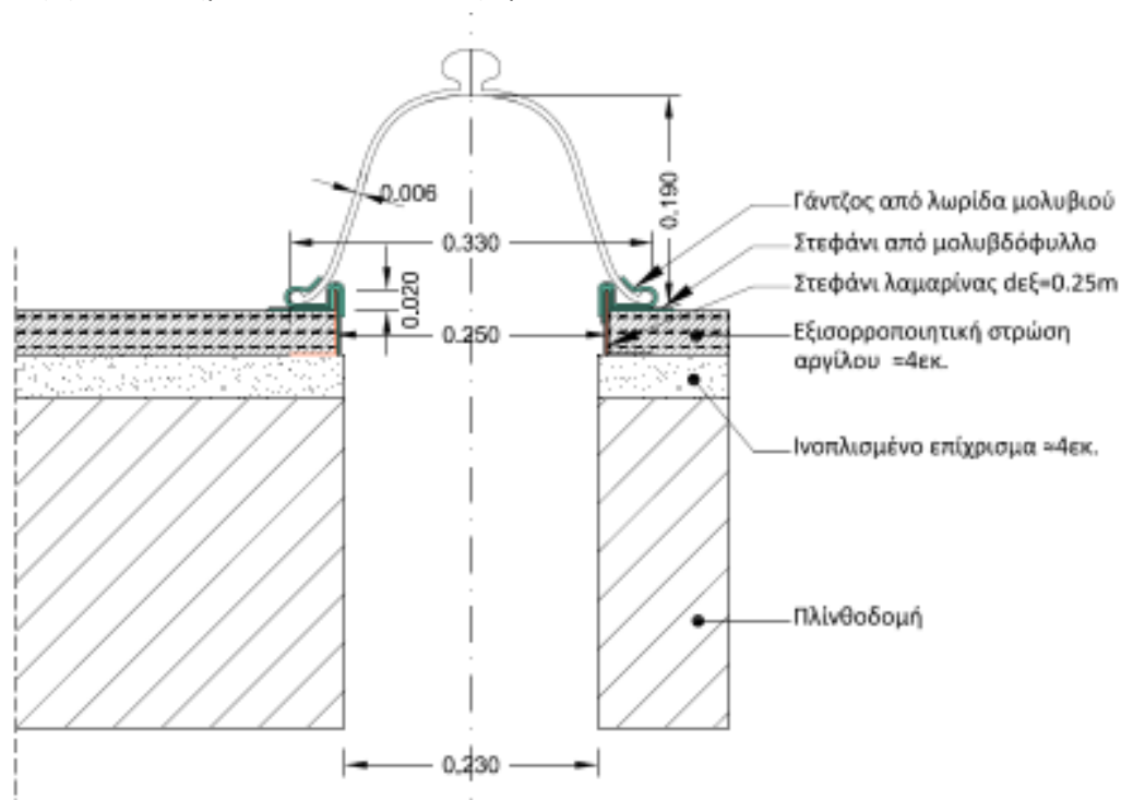
Εικόνα 4: Υάλινος κώδωνας (filgözü) τύπου Α
