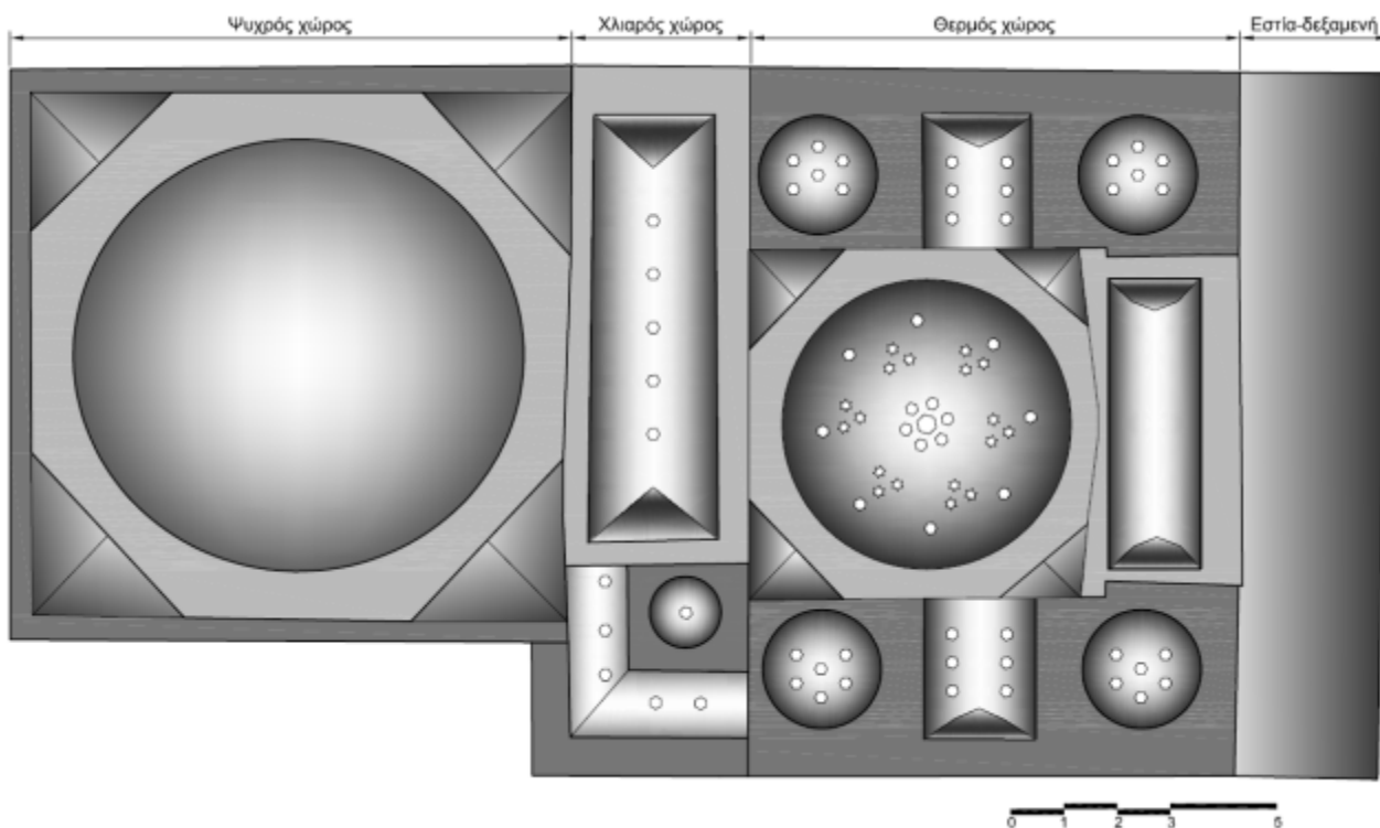
Εικόνα 1: Κάτοψη θολοδομίας Οθωμανικού Λουτρού στο Κάστρο Ιωαννίνων.
