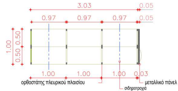
ΚΑΤΟΨΗ ΚΙΝΗΤΗΣ ΣΥΣΤΟΙΧΙΑΣ
