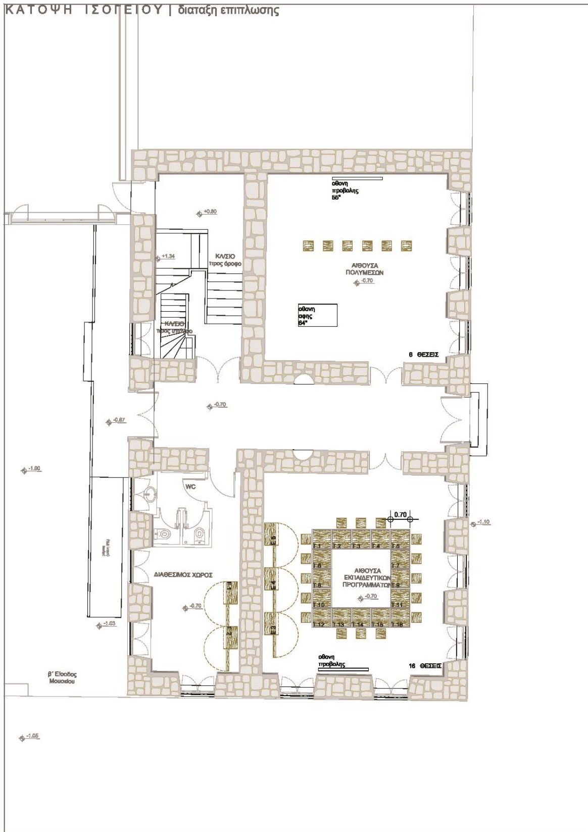
ΠΙΝ Α.01: κάτοψη ισογείου | χωροθέτηση εξοπλισμού
